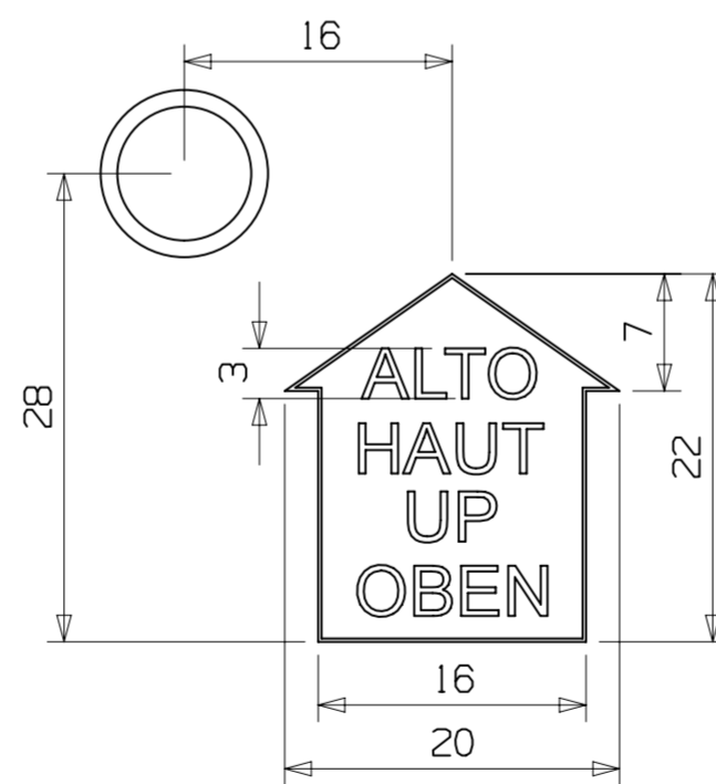
PARTICOLARE SCRITTE SCALA 2:1
